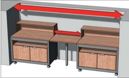
MODULO PER CONNESSIONE SU MISURA CUSTOMIZED CONNECTION MODULE Spesso gli spazi disponibili non sono perfettamente compatibili con le dimensioni standard del Break. Nel caso, Opt. L e Opt. ANG possono essere personalizzati/modificati in base ai tuoi bisogni. Often the spaces available are not perfectly compatible with the standard dimensions of the Break. In case, Opt.L and Opt.ANG can be customized / modified according to your needs.
